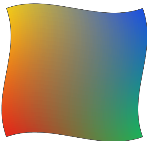
Un carreau de Coons : quatre côtés courbes
