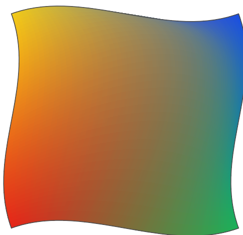
Un carreau tensoriel, tiré de l'intérieur
