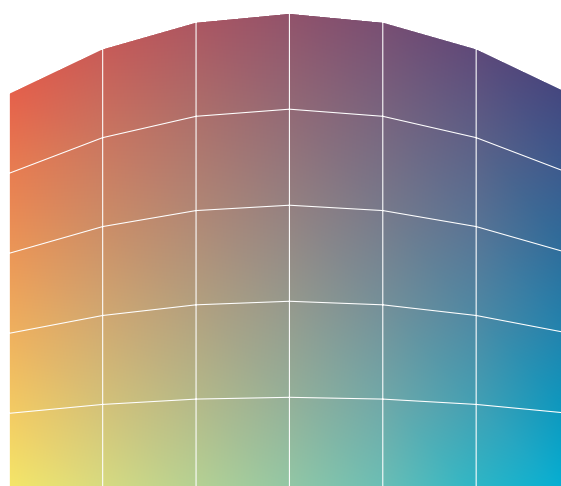
Un treillis de points, en quatre encres
